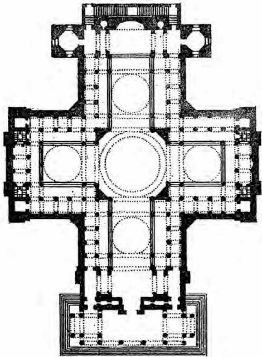
J.-G. Soufflot, Sainte-Geneviève, 1764-1790; pianta dopo i restauri del 1806-1812 (da A.-Ch. Quatremère de Quincy, Histoire de la vie et des ouvrages... , Paris, 1830)
