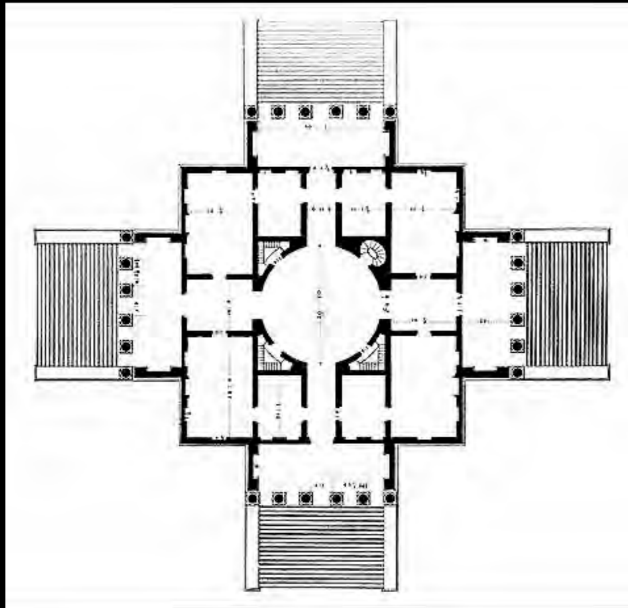
Andrea Palladio : Villa Capra, Vicenza, 1566 - Planta de "i quattri libri" - (1570) - Publicacion de Scamozzi, 1778
